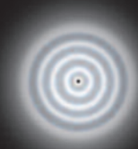
Intra-focale (rifrattore)
